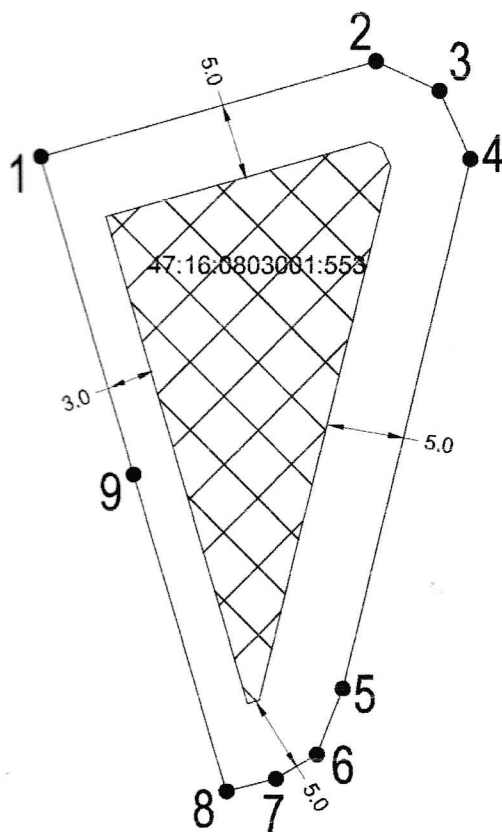
СИТУАЦИОННЫЙ ПЛАН
